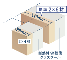
2×4材より断熱層を厚くできる2×6材を使用。
